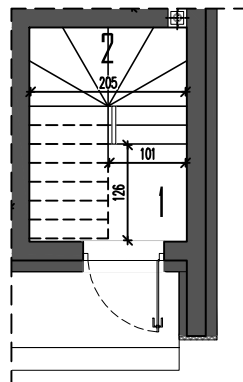
RZUT PARTERU
