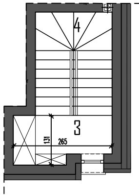
RZUT PIĘTRA
